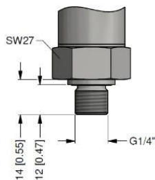
G1/4" DIN 3852
