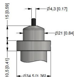
dławnica kablowa PG7 / należy podać długość kabla (IP 67) 6
