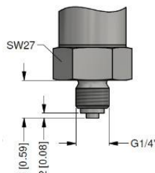
G1/4" EN 837
