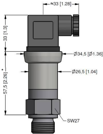
G1/2" DIN 3852 / ISO 4400
